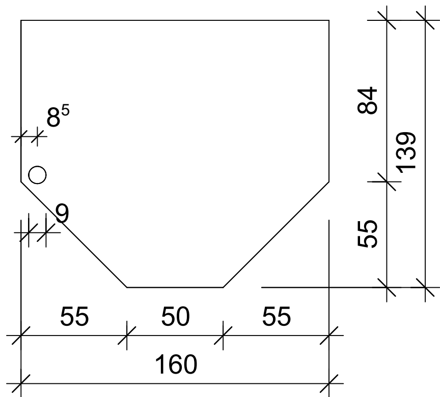
Ansicht 1-1, 1:2
