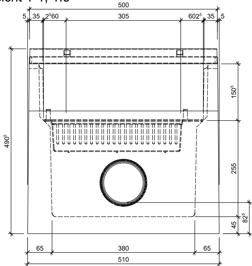
Ansicht 1-1, 1:5
