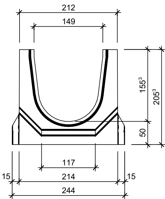
Schnitt 2-2, 1:5 Feder
