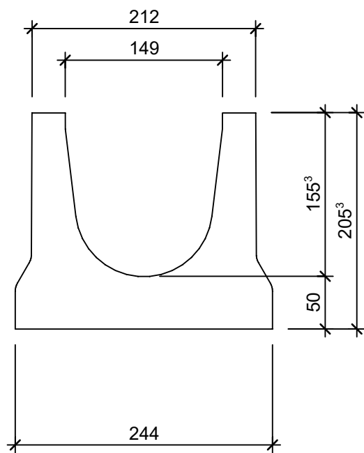
Schnitt 3-3, 1:5 Nut
