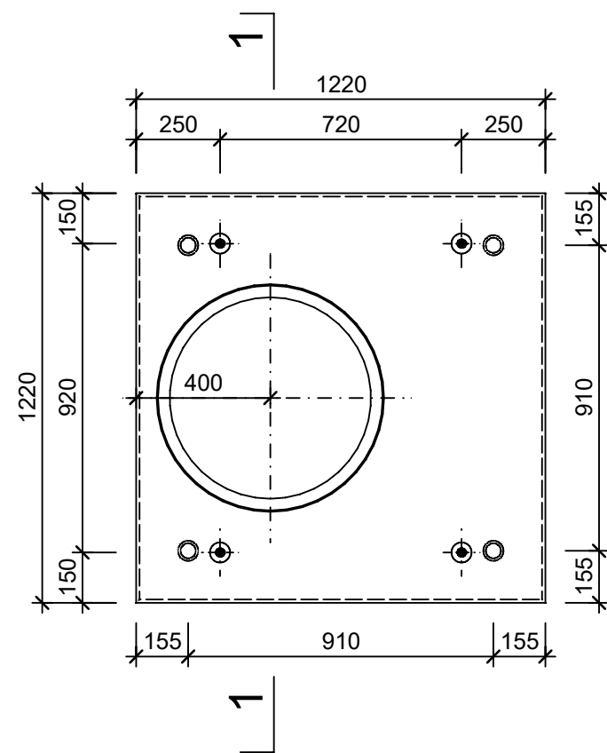
Grundriss, 1:20
