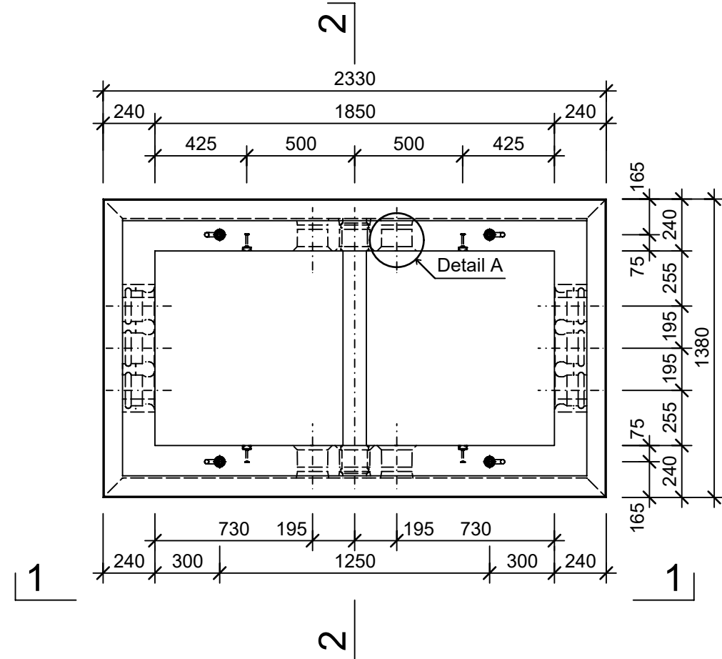
Grundriss, 1:25
