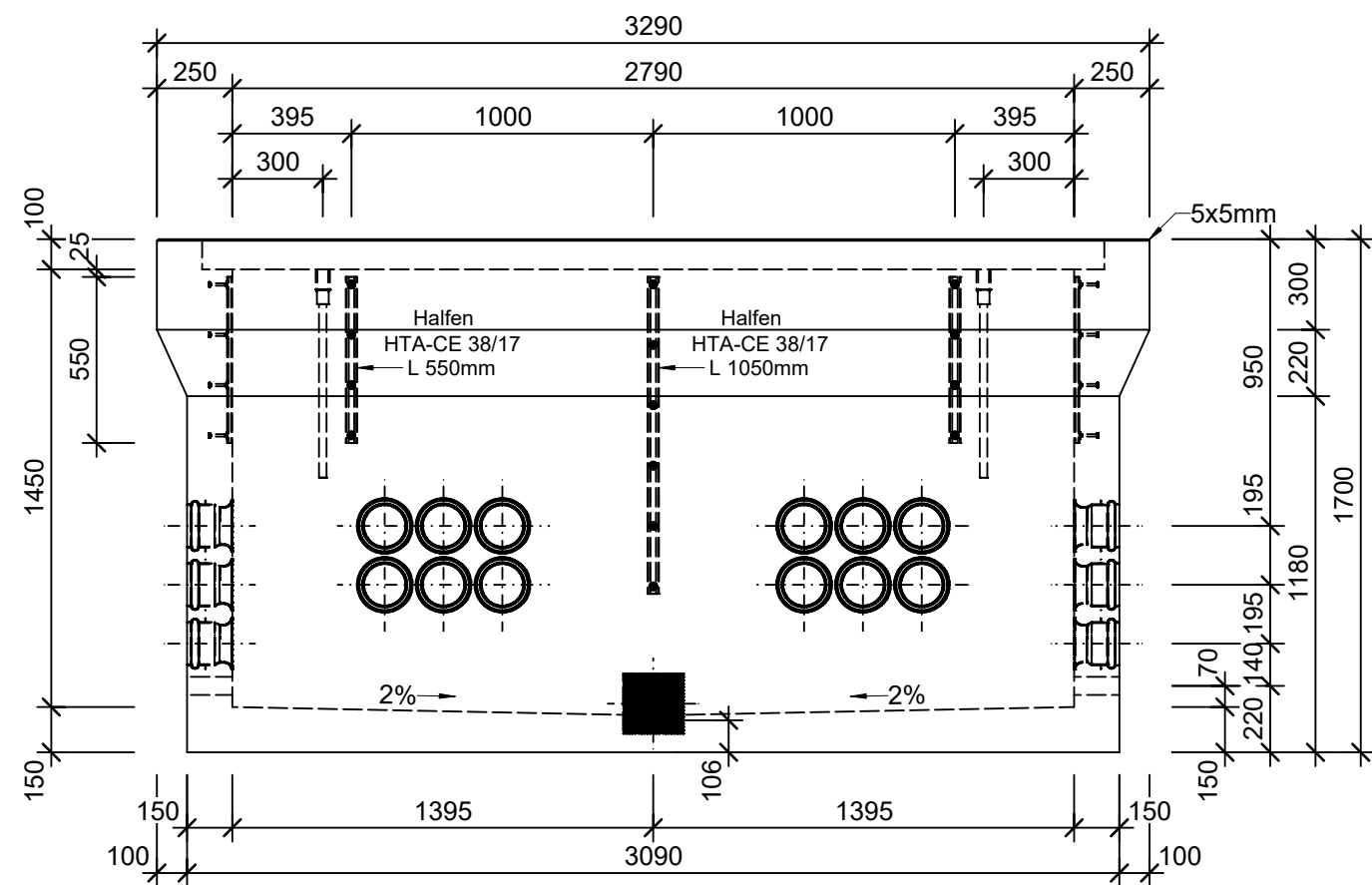
Grundriss, 1:25
