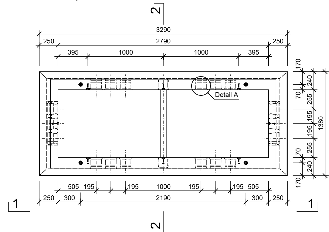
Grundriss, 1:25
