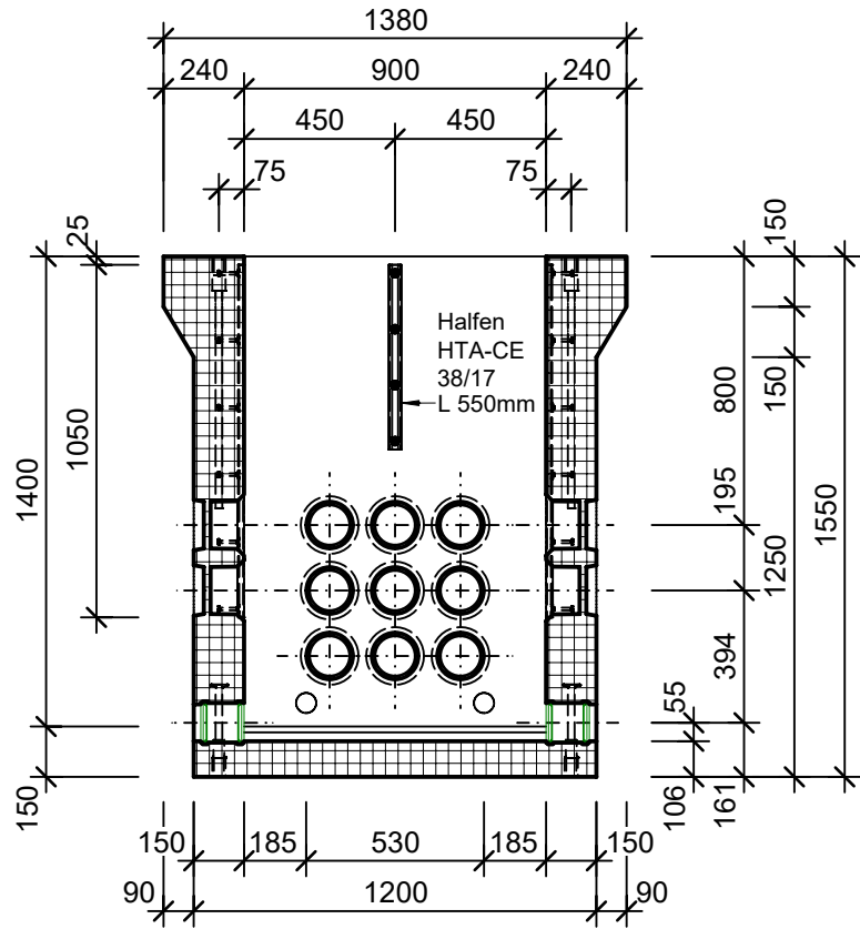
Schnitt 2-2, 1:25
