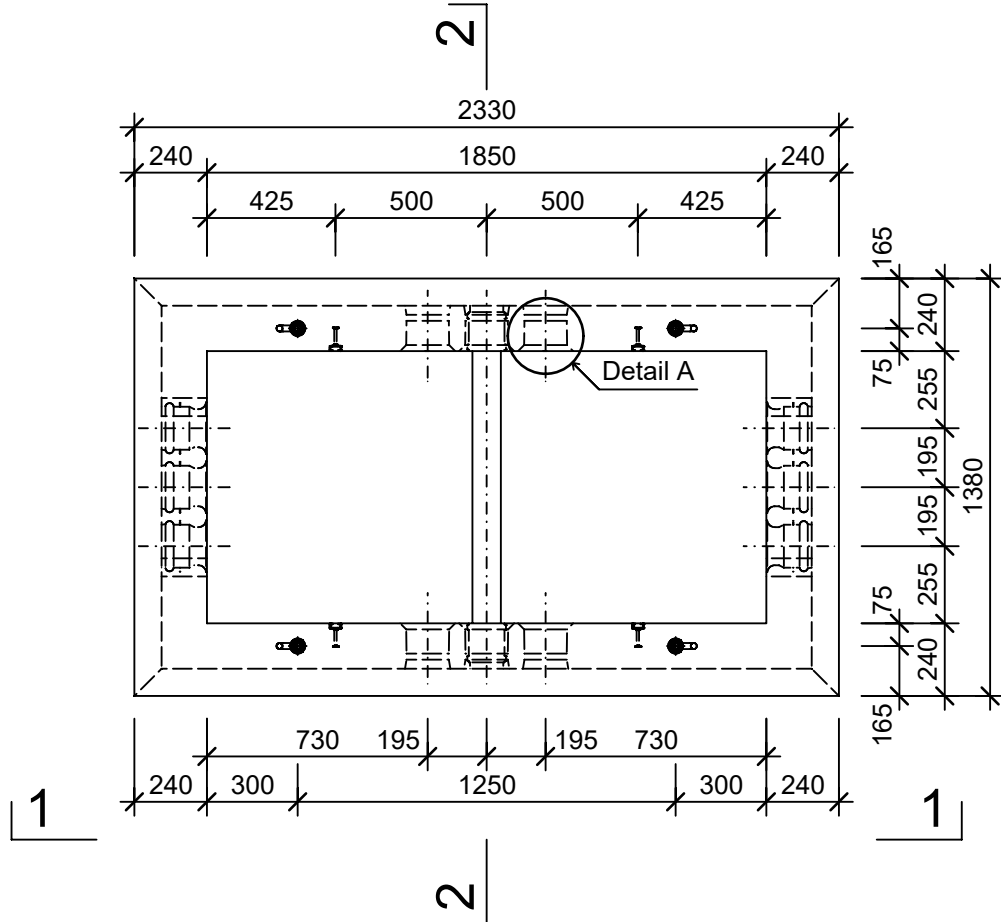
Grundriss, 1:25
