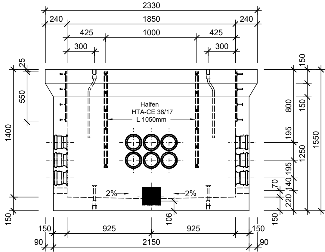
Ansicht 1-1, 1:25
