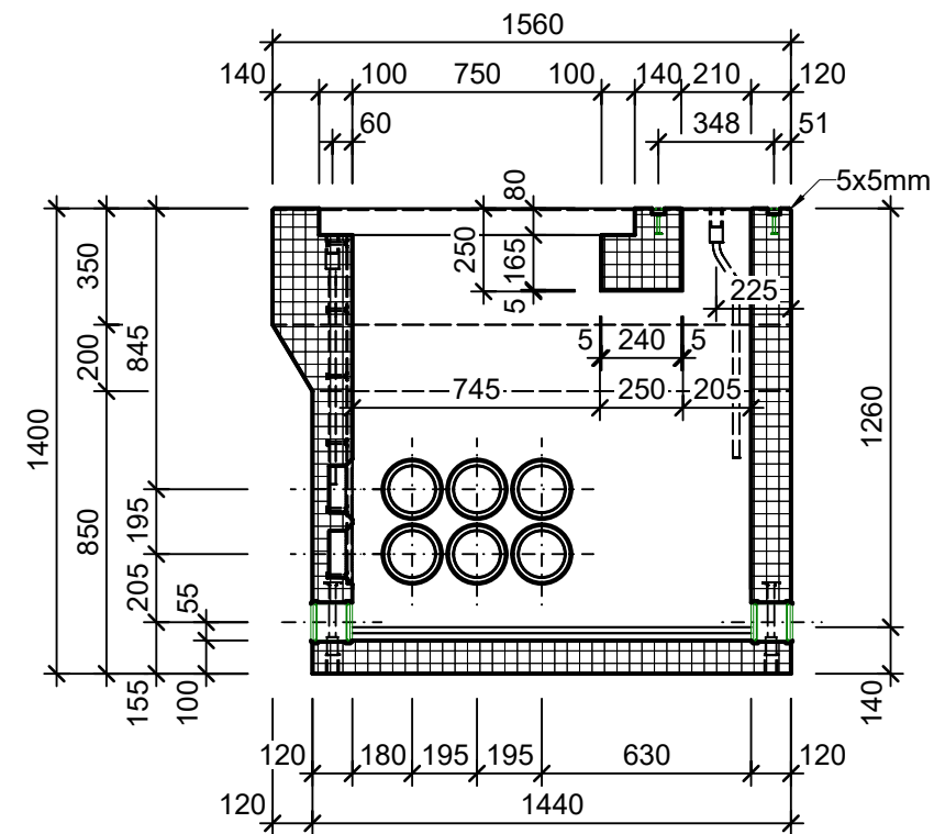
Schnitt 2-2, 1:25
