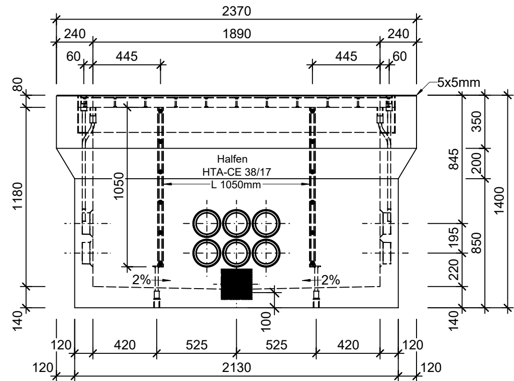
Ansicht 1-1, 1:25
