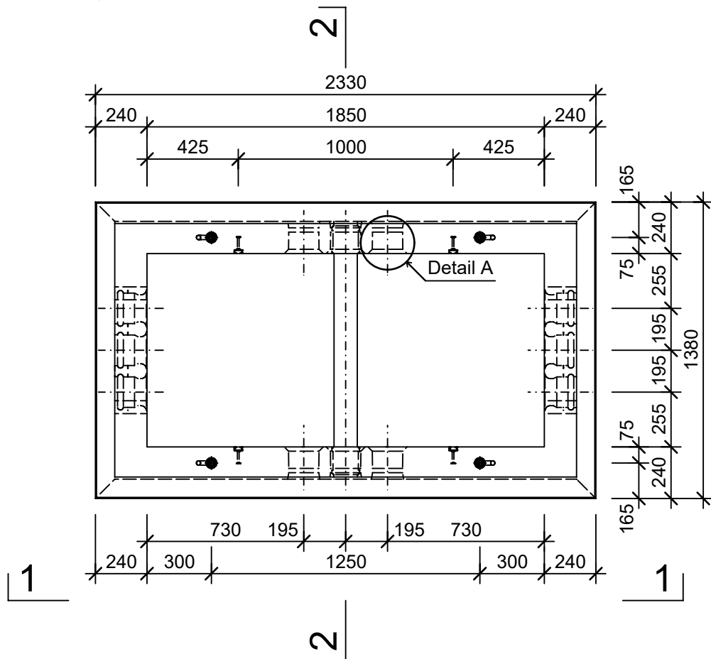
Grundriss, 1:25
