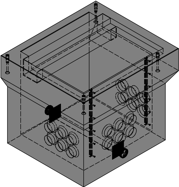
Isometrie
