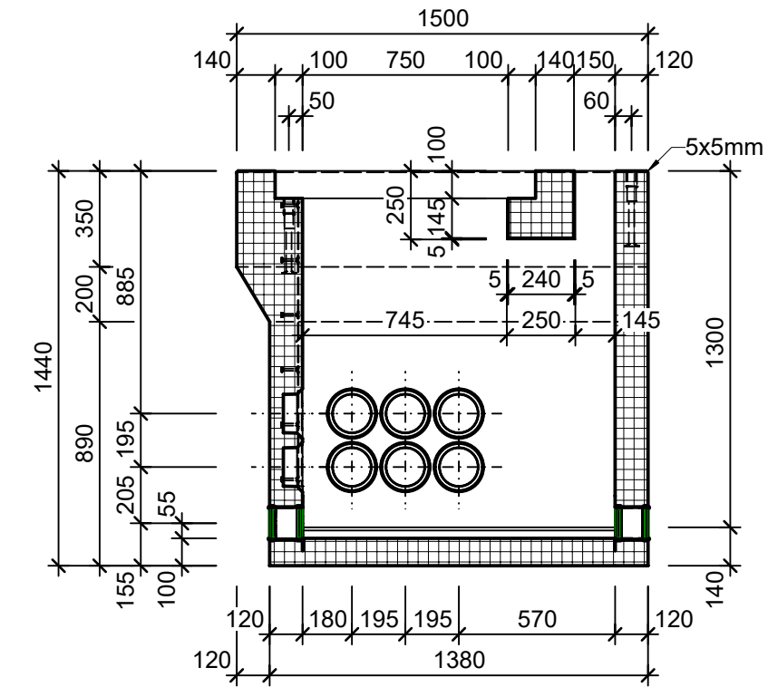
Schnitt 2-2, 1:25
