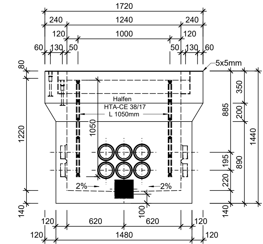
Ansicht 1-1, 1:25
