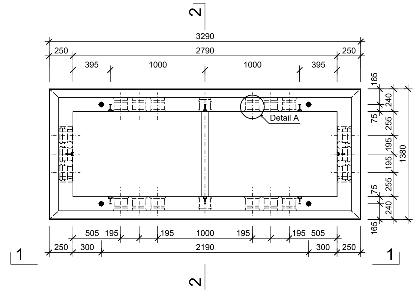
Grundriss, 1:25
