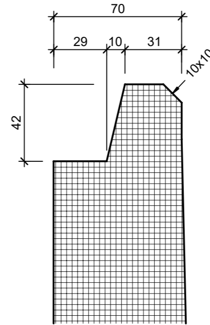
Detail A, 1:2
