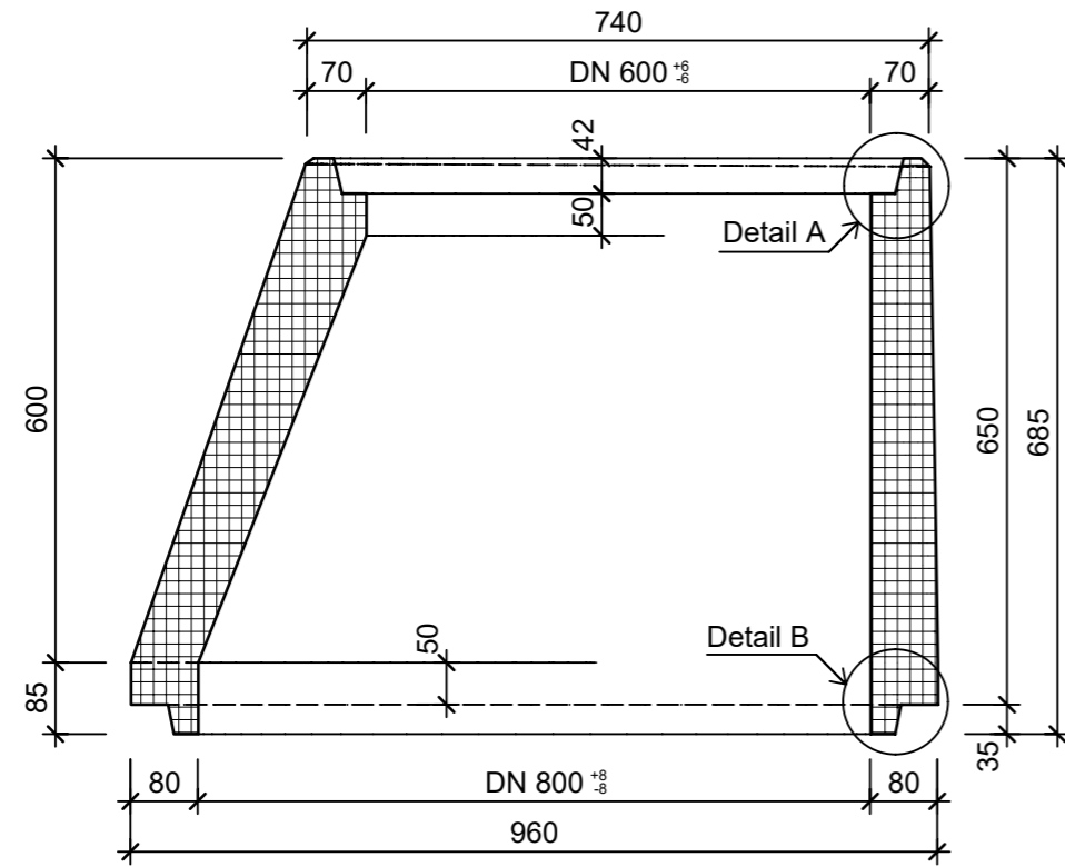
Ansicht 1-1, 1:10
