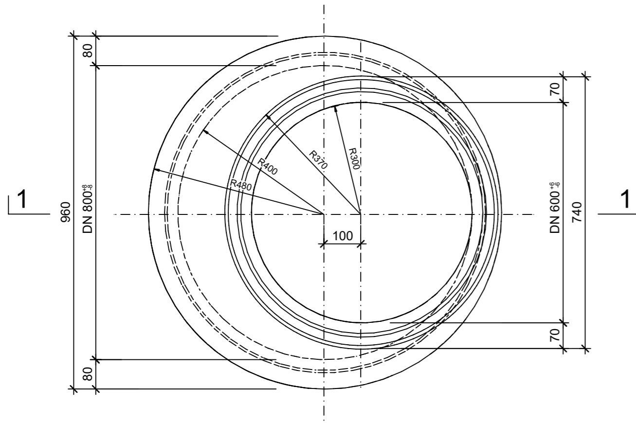
Grundriss, 1:10
