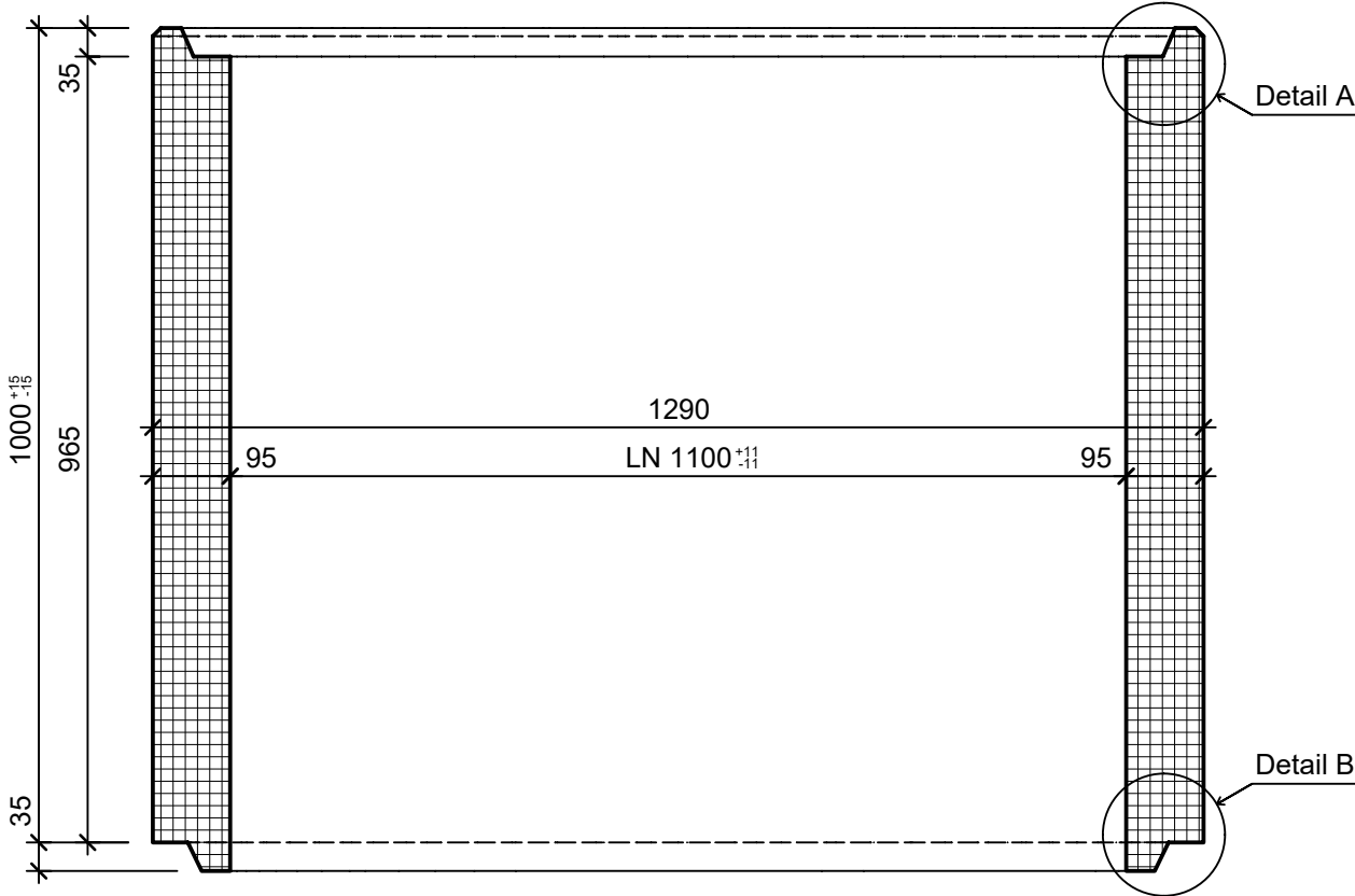
Grundriss, 1:10
