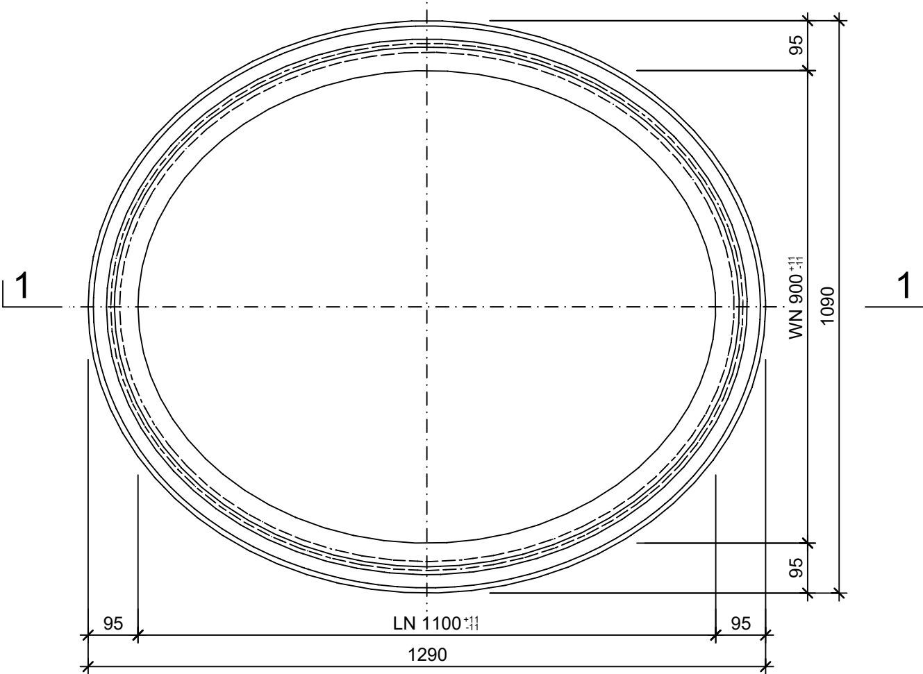
Grundriss, 1:10
