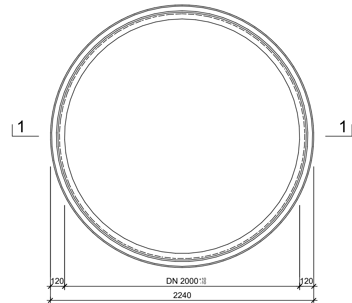
Grundriss, 1:20
