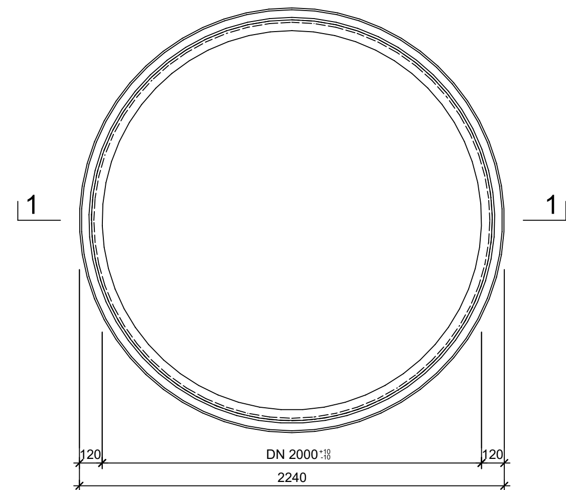
Grundriss, 1:20
