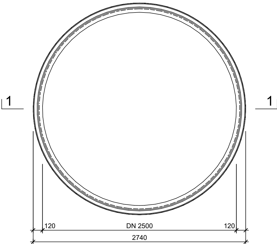
Grundriss, 1:25
