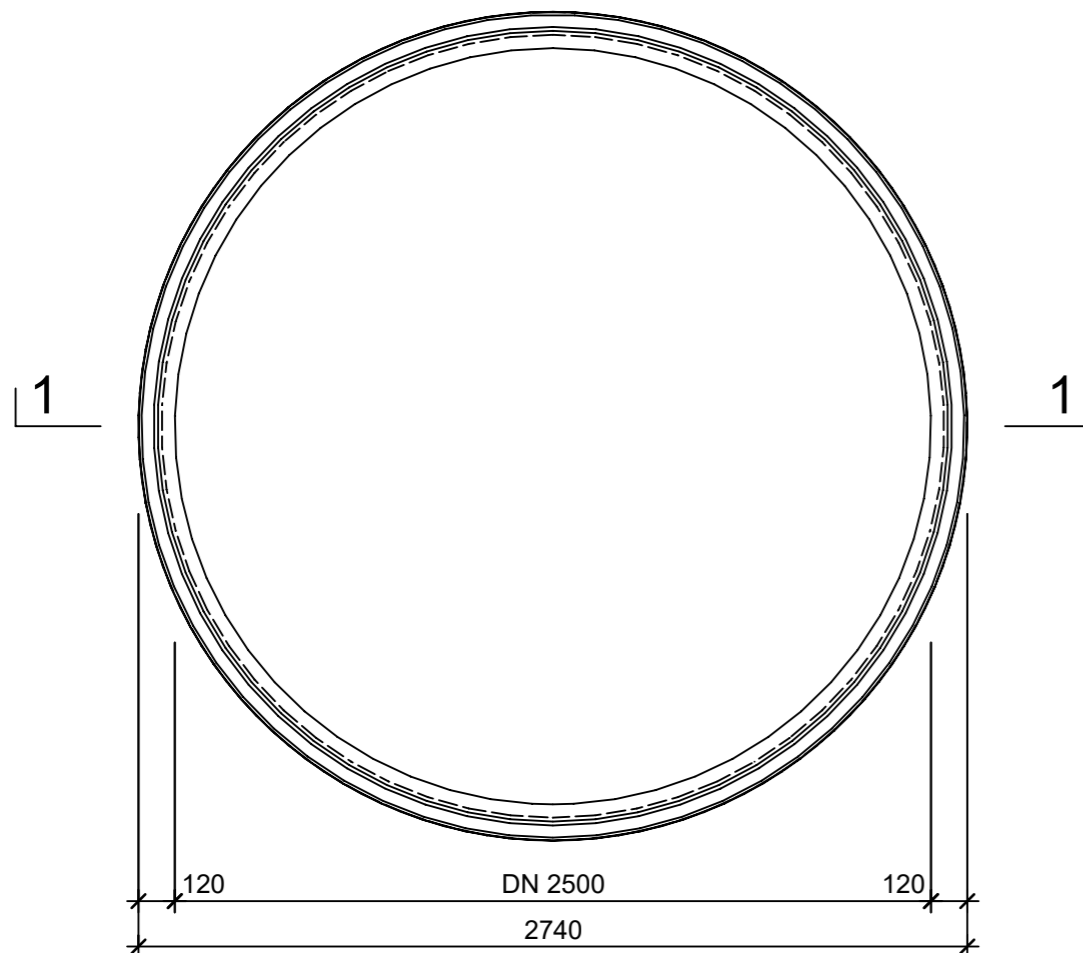
Grundriss, 1:25
