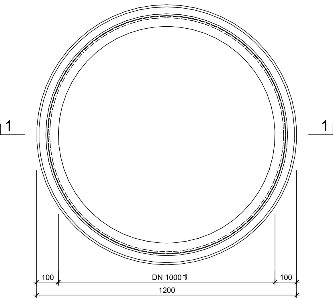
Grundriss, 1:10
