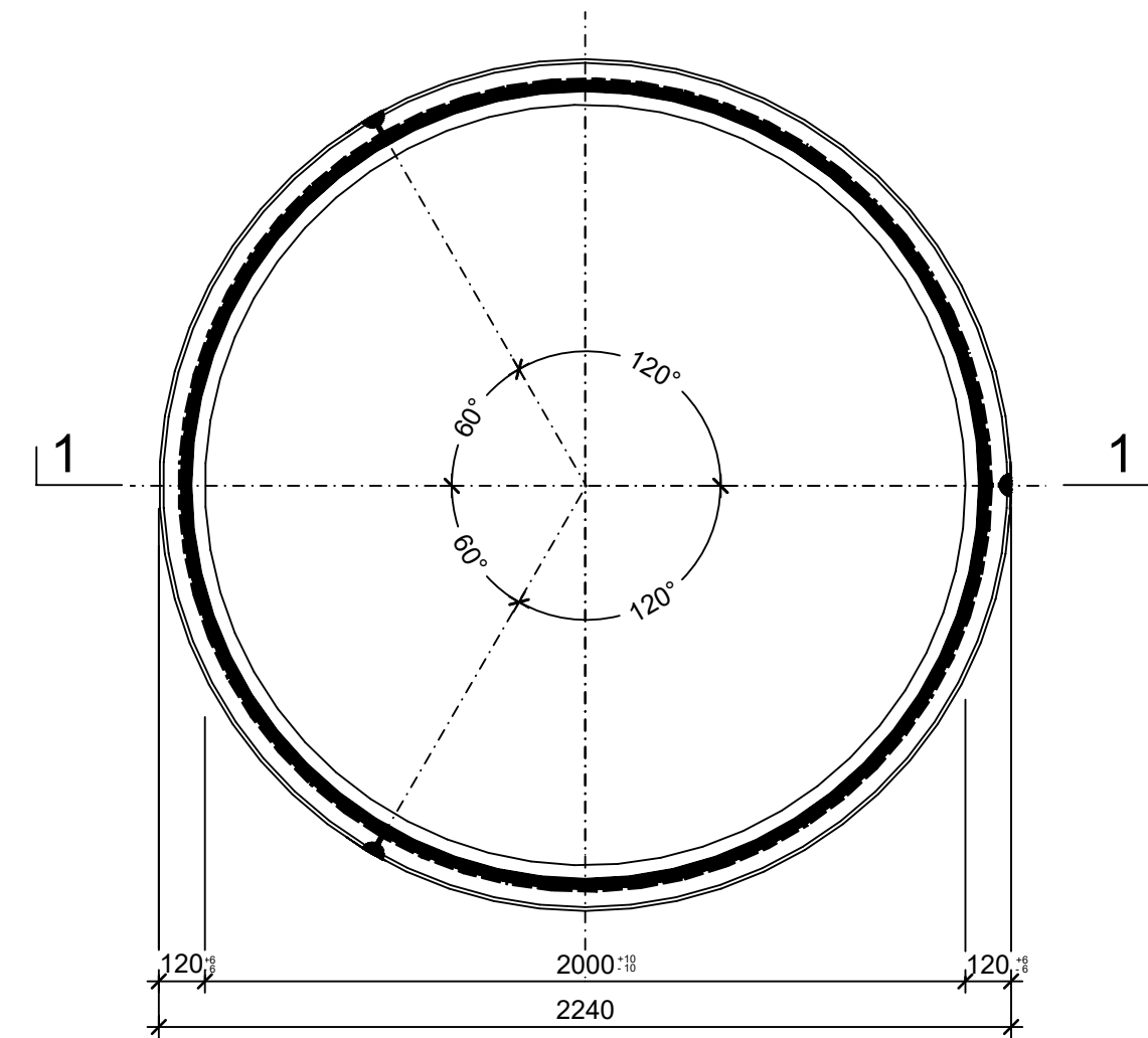
Grundriss, 1:20
