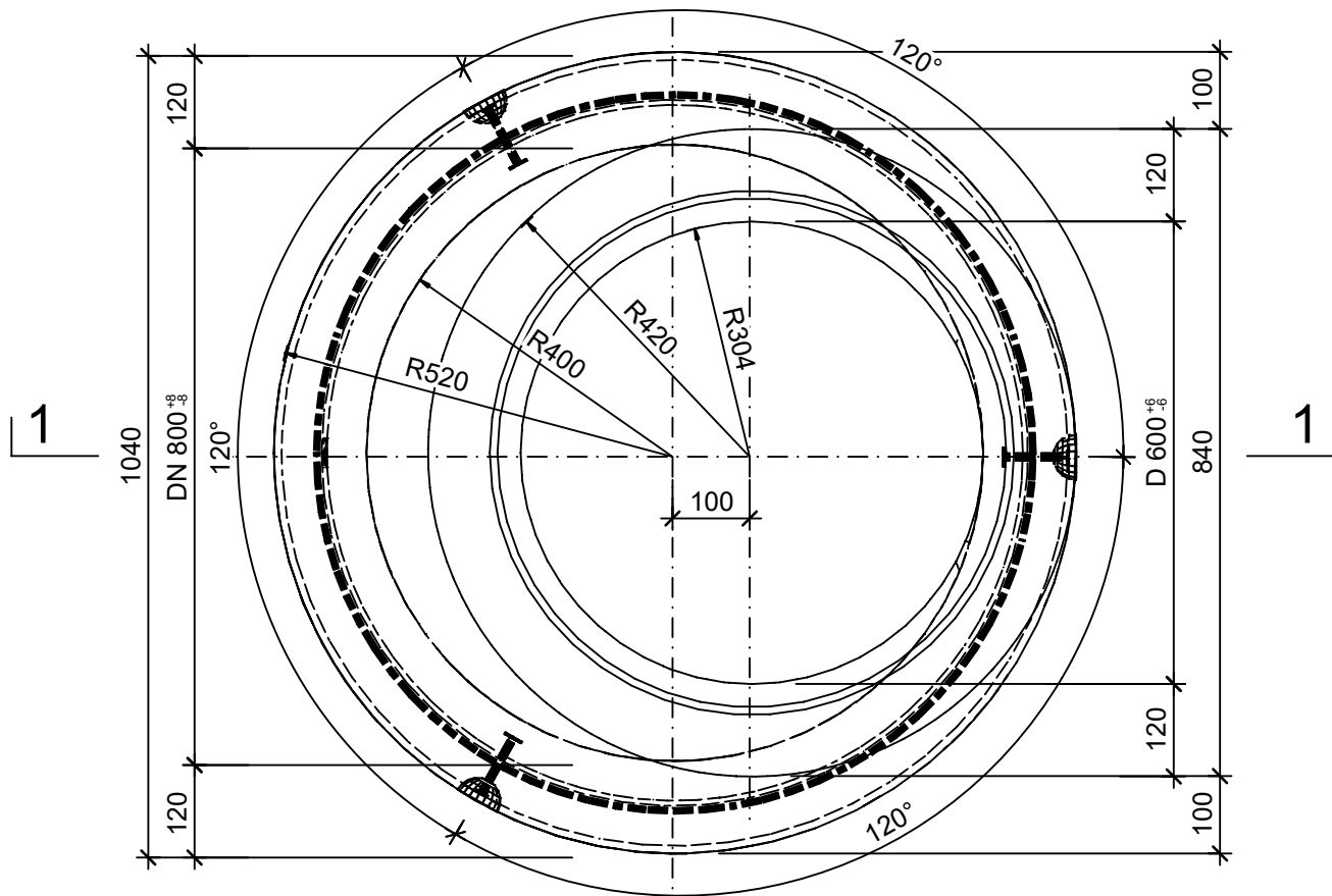
Grundriss, 1:10
