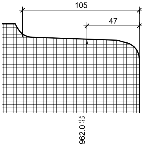
Detail Spitzende, 1:2
